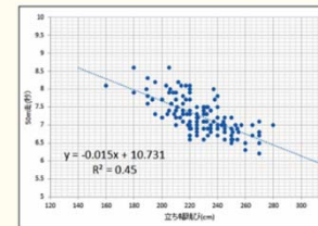
図表5 立ち幅跳び(X)と50m走のタイム(Y)の散布図と予測式 出典：「情報1」 教育研究用教材 より引用
